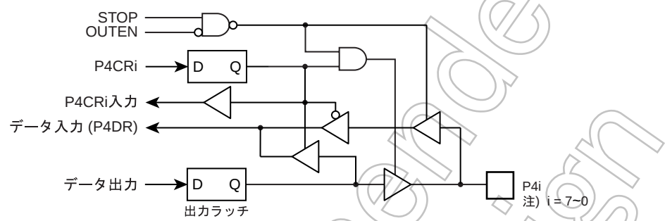
図 5-6 P4 ポート
