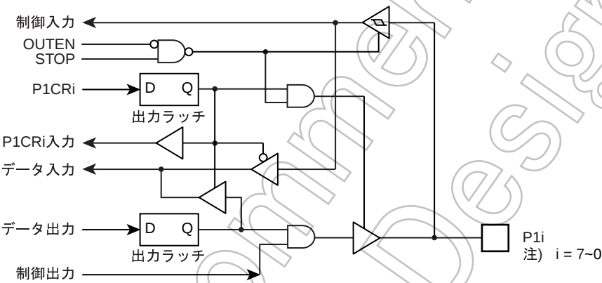
図 5-3 P1 ポート
