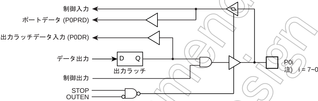
図 5-2 P0 ポート
