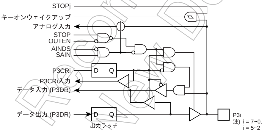
図 5-5 P3 ポート
