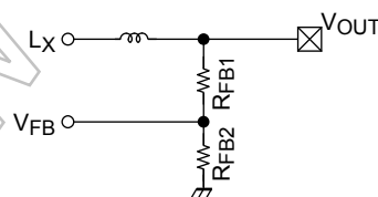
図 3 出力電圧設定抵抗
