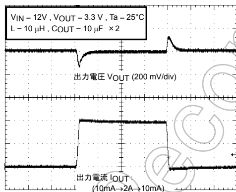
負荷応答特性
