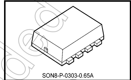
SON8-P-0303-0.65A 質量: 0.017 g (標準)
