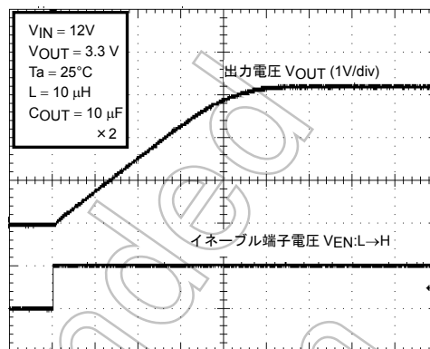
起動特性 ( C_{SS} = 0.1\mu\text{F} )
