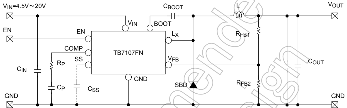
図 1 TB7107FN 応用回路例
