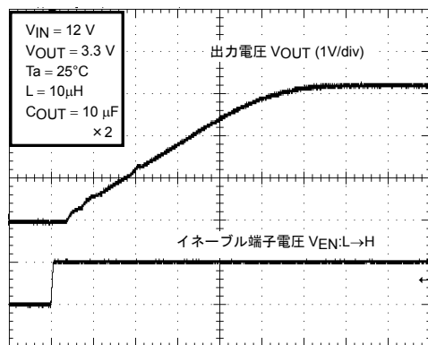
起動特性 (内部ソフトスタート時間)
