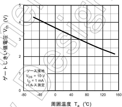
図 8.10 V_{th} - T_a
