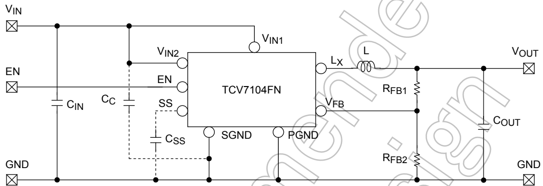
図 1 TCV7104FN 応用回路例
