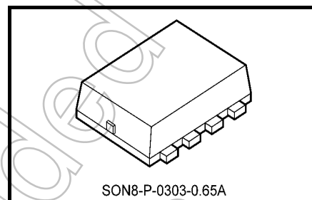
SON8-P-0303-0.65A 質量: 0.017 g (標準)
