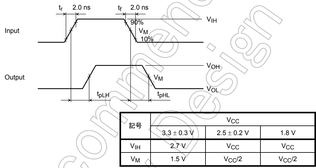
図 2 t_{pLH} , t_{pHL}
