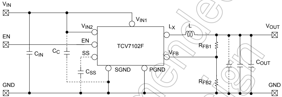
図 1 TCV7102F 応用回路例
