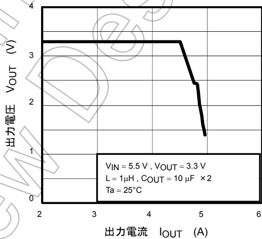
過電流特性
