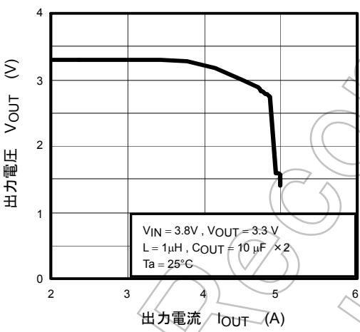
過電流特性
