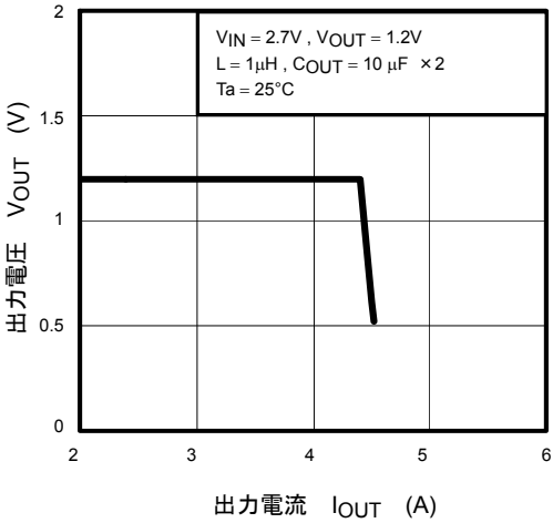
過電流特性
