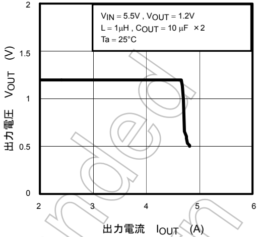
過電流特性
