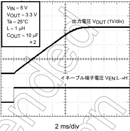
起動特性 ( C_{SS} = 0.1\text{ }\mu\text{F} )
