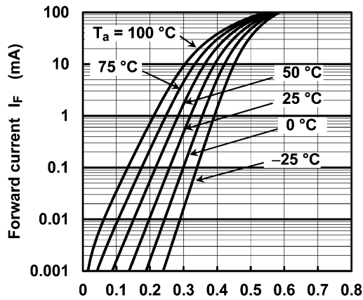
Fig. 8.1 I_F - V_F
