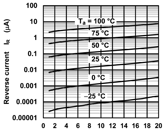
Fig. 8.2 I_R - V_R
