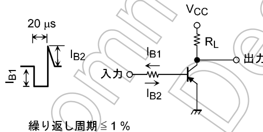
図 6.2.1 スwitchング時間の測定回路
