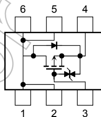
内部接続 (top view)
