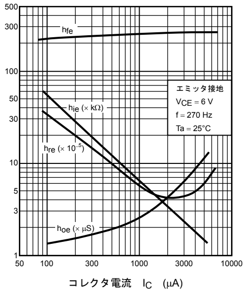
h パラメータ - I_C
