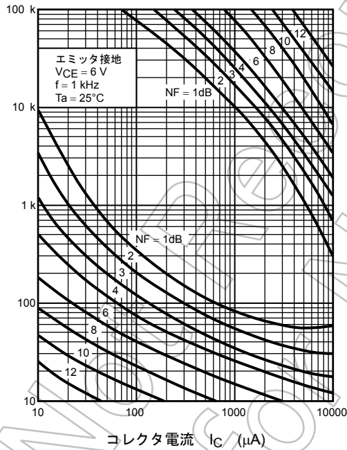
NF - R_G, I_C
