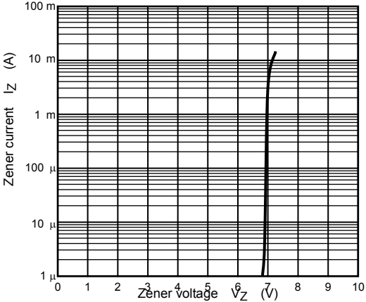
I_Z - V_Z
