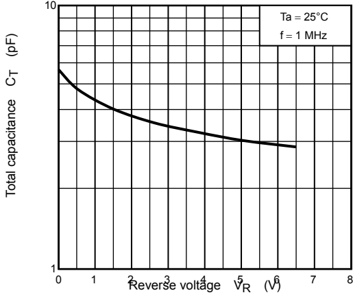
C_T - V_R
