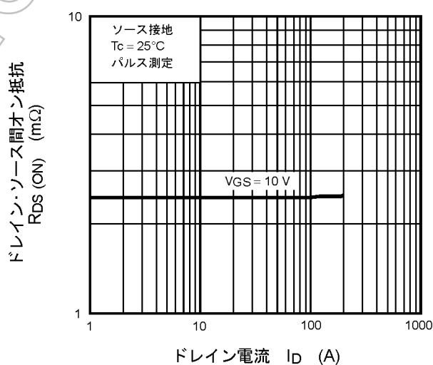
図 9.6 R_{DS(ON)} - I_D
