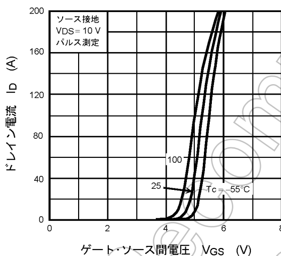
図 9.3 I_D - V_{GS}
