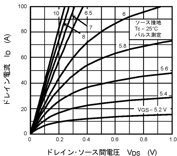
図 9.1 I_D - V_{DS}
