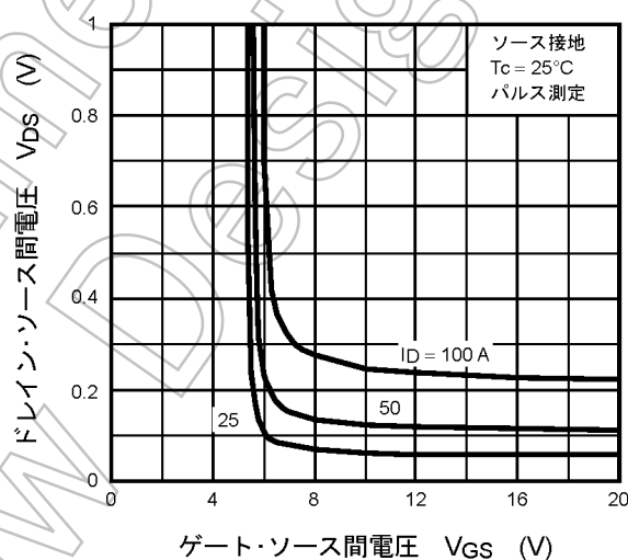
図 9.4 V_{DS} - V_{GS}
