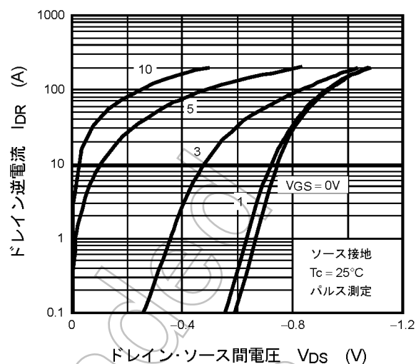
図 9.8 I_{DR} - V_{DS}
