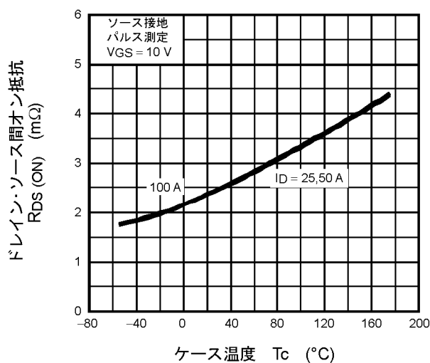
図 9.7 R_{DS(ON)} - T_c
