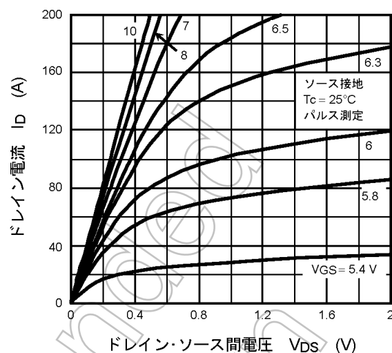
図 9.2 I_D - V_{DS}
