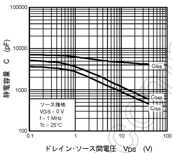
図 9.9 静電容量 - V_{DS}
