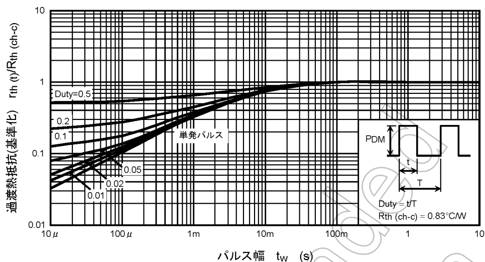
図 9.13 r_{th}/R_{th(ch-c)} - t_w (最大値 (保証値))
