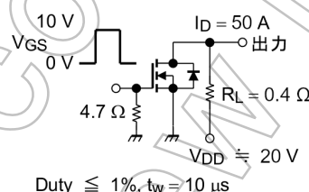
図 6.2.1 スwitchング時間の測定回路
