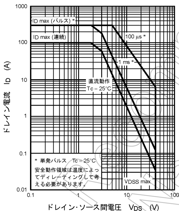
図 9.14 安全動作領域 (最大値 (保証値))
