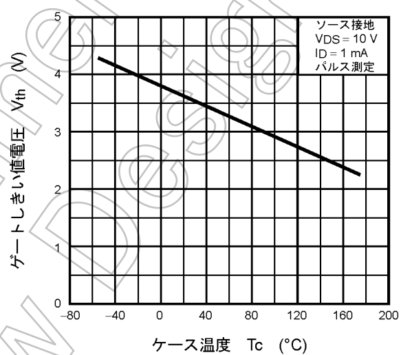
図 9.10 V_{th} - T_c
