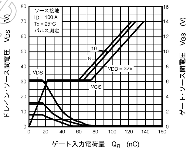
図 9.12 ダイナミック入出力特性
