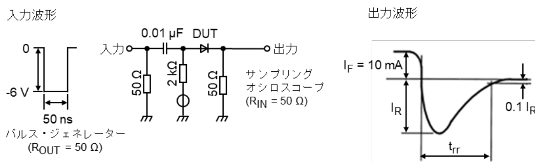
図 1. 逆回復時間 ( t_{rr} ) 測定回路
