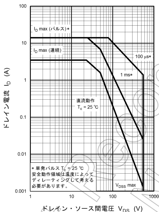
図 8.14 安全動作領域 (最大値 (保証値))
