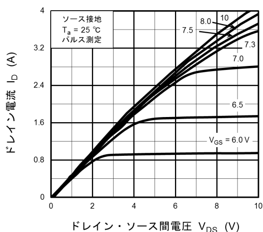
図 8.1 I_D - V_{DS}
