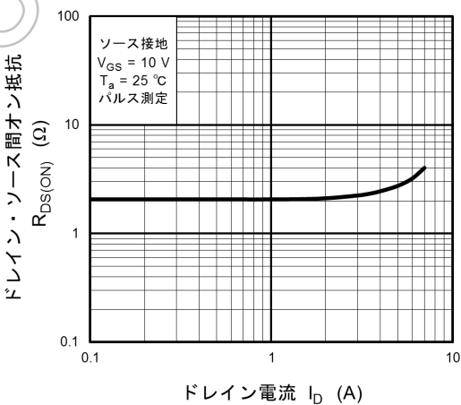
図 8.6 R_{DS(on)} - I_D
