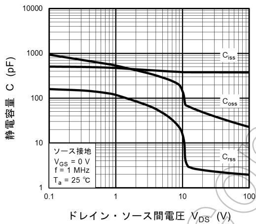
図 8.9 C - V_{DS}
