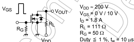
図 6.2.1 スwitchング時間の測定回路例
