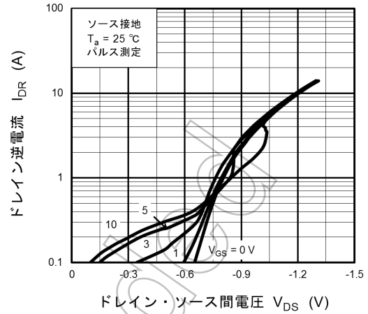
図 8.8 I_{DR} - V_{DS}
