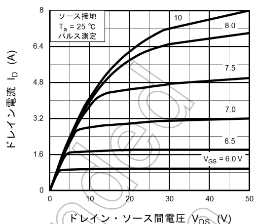
図 8.2 I_D - V_{DS}
