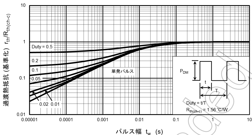
図 8.13 r_{tr}/R_{th(ch-c)} - t_w (最大値 (保証値))
