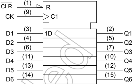
論理図
