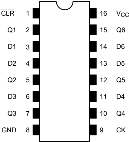
ピン接続図 (top view)
