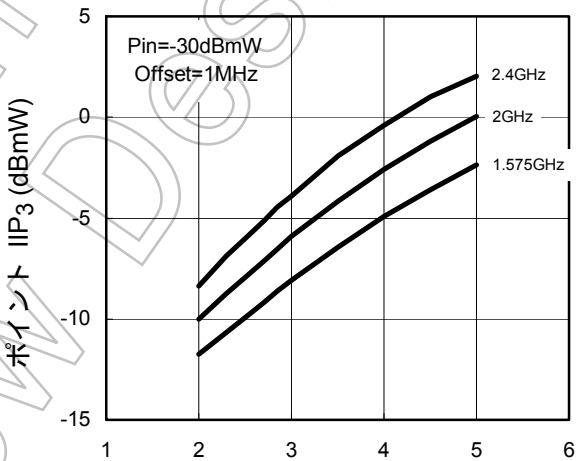
電源電圧 V CC (V)
