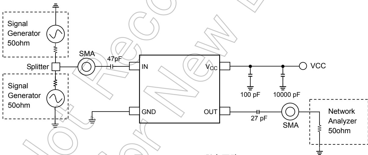
図 3 . OIP3 , IIP3 測定回路
