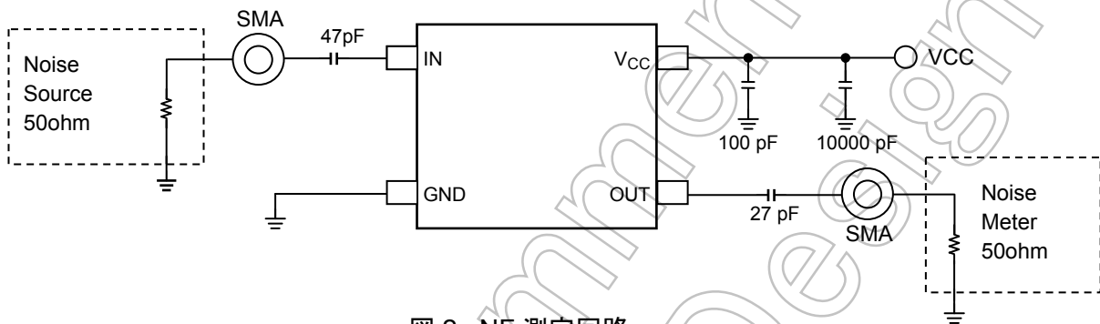
図 2 . NF 測定回路
