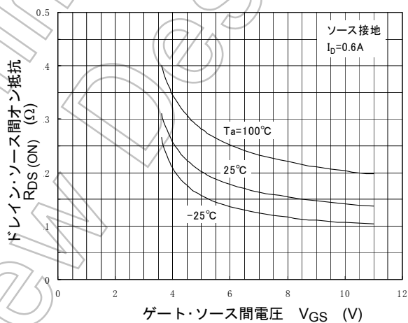
R_{DS(ON)} - V_{GS}
