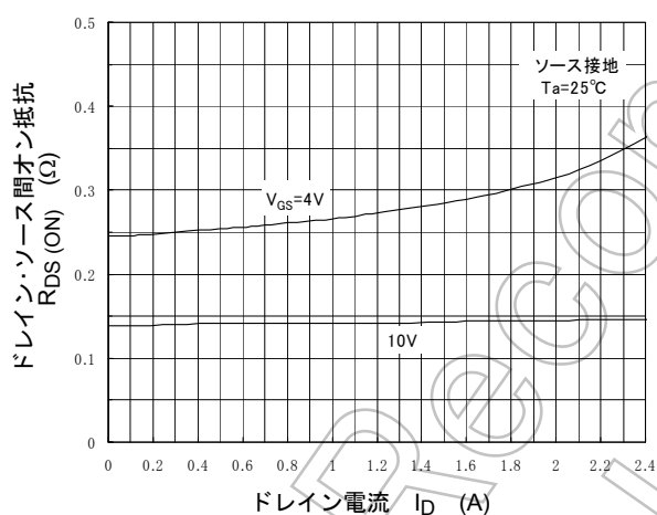
R_{DS(ON)} - I_D
