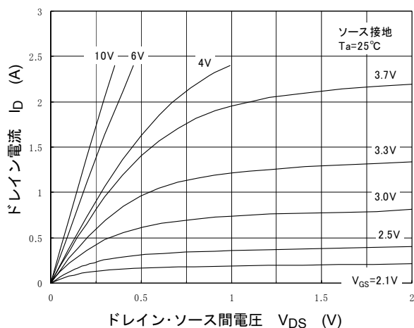
I_D - V_{DS}
