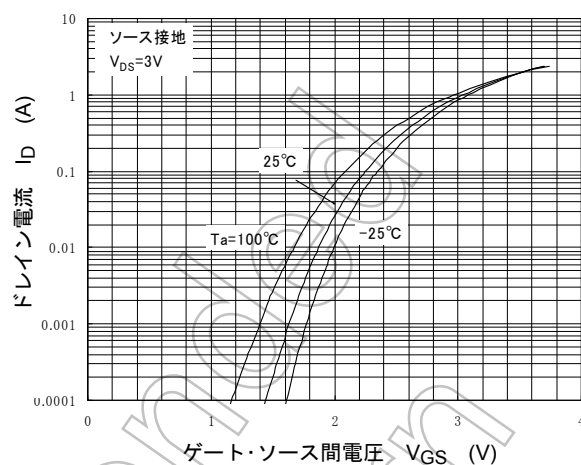
I_D - V_{GS}
