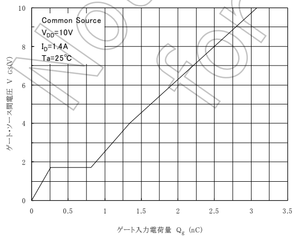
ダイナミック入力特性
