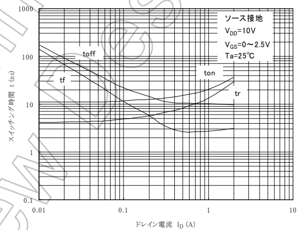
t - I_D
