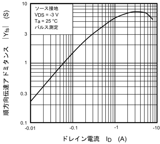
図 8.7 |Y_{fs}| - I_D
