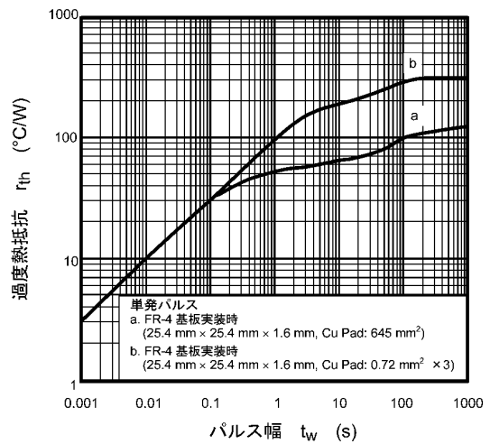
図 8.12 r_{th} - t_w
