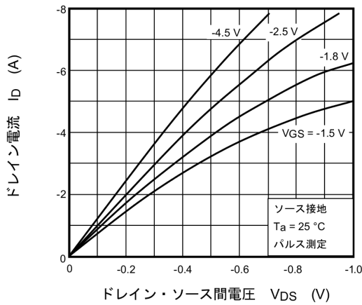
図 8.1 I_D - V_{DS}
