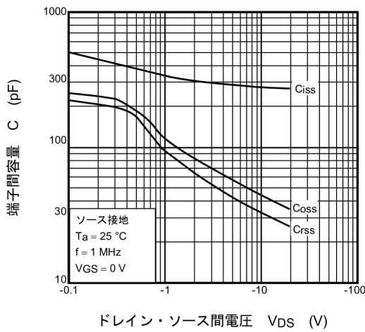
図 8.9 C - V_{DS}
