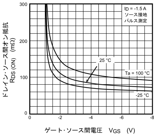
図 8.3 R_{DS(ON)} - V_{GS}
