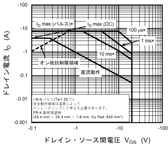
図 8.14 安全動作領域
