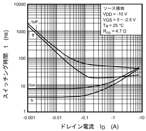
図 8.10 t - I_D
