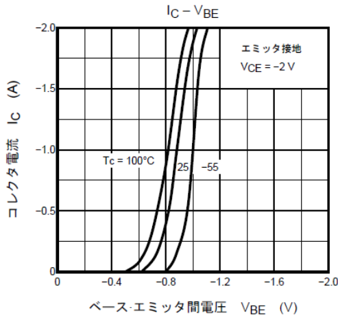
図 8.7 I_C - V_{BE}
