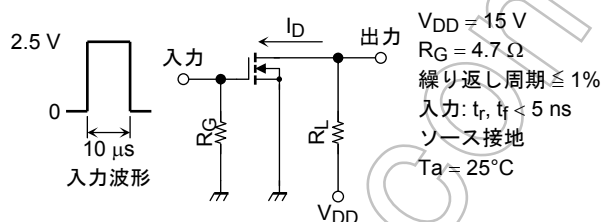
(a) 測定回路
