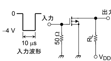
(a) 測定回路
