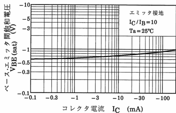
図 13.4 V_{BE(sat)} - I_C
