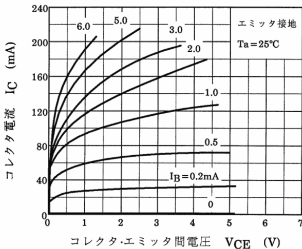
図 14.1 I_C - V_{CE}
