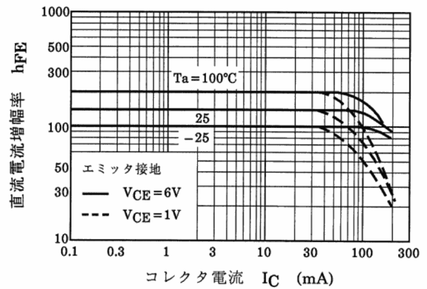
図 14.2 h_{FE} - I_C
