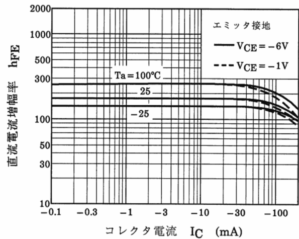
図 13.2 h_{FE} - I_C
