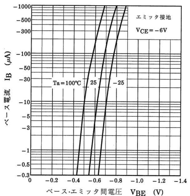
図 13.6 I_B - V_{BE}
