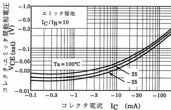
図 13.3 V_{CE(sat)} - I_C
