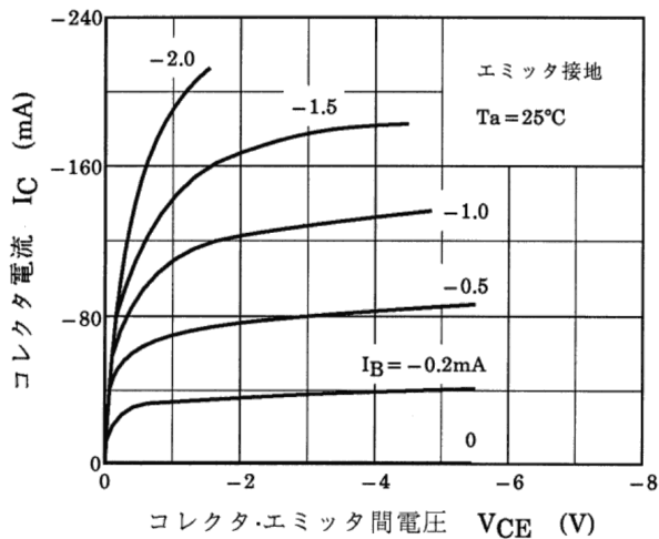
図 13.1 I_C - V_{CE}
