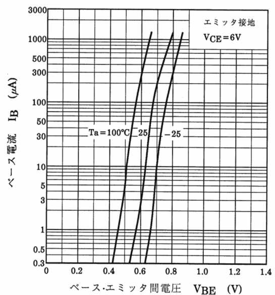
図 14.6 I_B - V_{BE}
