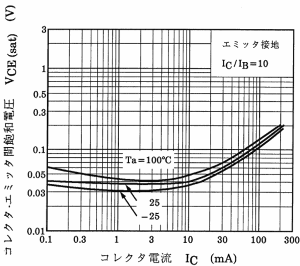
図 14.3 V_{CE(sat)} - I_C
