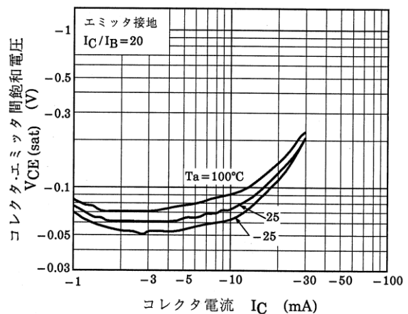
図 7.11 RN2709JE V_{CE(sat)} - I_C
