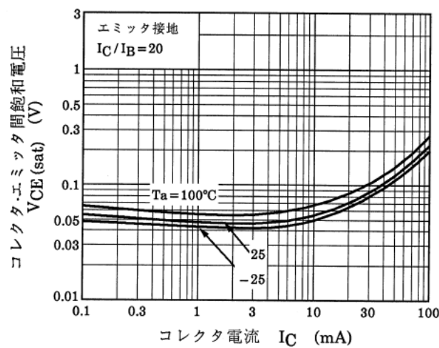
図 9.8 RN1911FE V_{CE(sat)} - I_C
