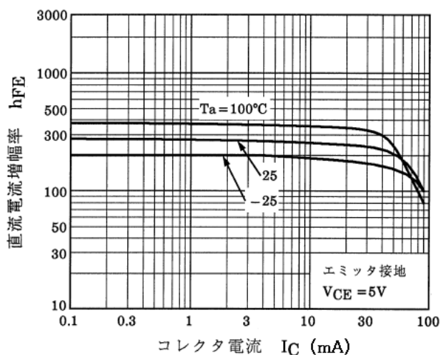
図 9.5 RN1910FE h_{FE} - I_C
