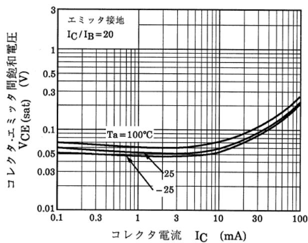
図 9.7 RN1910FE V_{CE(sat)} - I_C
