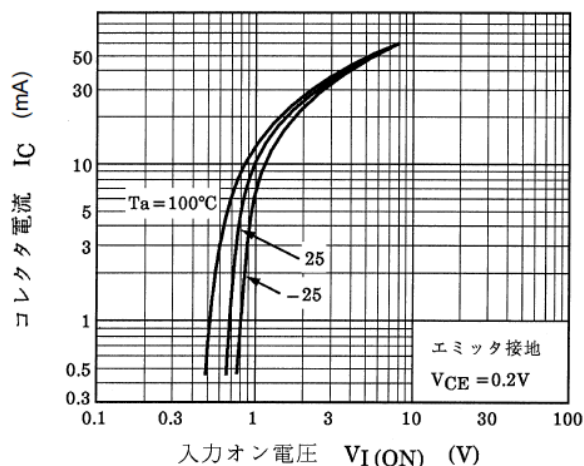
図 9.1 RN1910FE I_C - V_{I(ON)}
