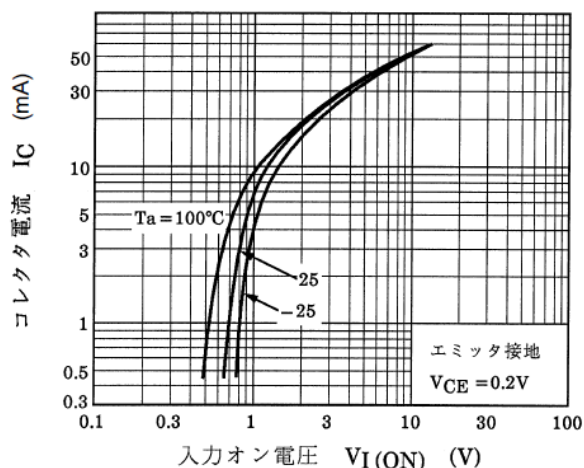
図 9.2 RN1911FE I_C - V_{I(ON)}
