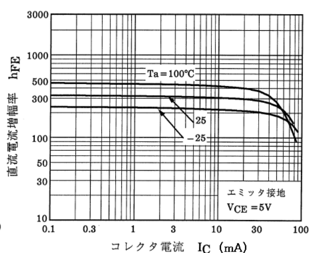
図 9.6 RN1911FE h_{FE} - I_C
