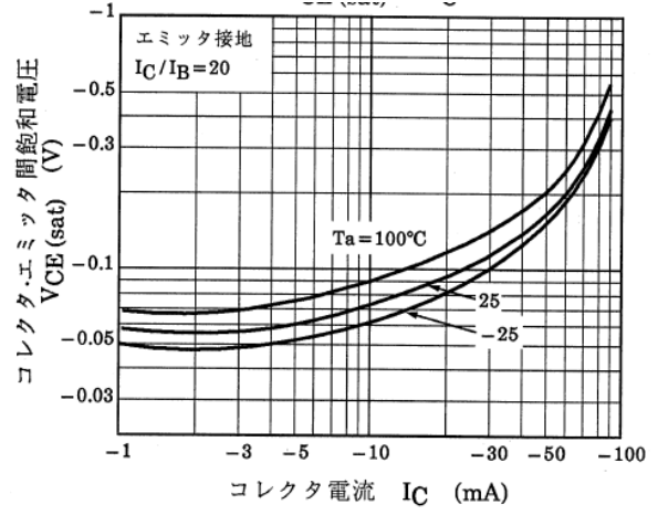
図 13.8 Q2 V_{CE(sat)}-I_C
