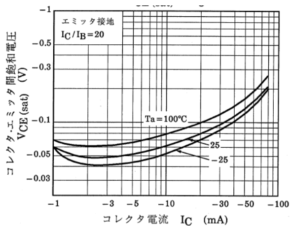
図 13.8 Q2 VCE(sat)-IC
