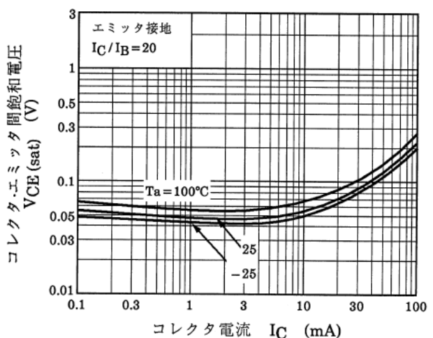
図 13.8 Q2 V_{CE(sat)}-I_C
