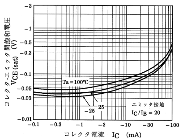
図 13.7 Q1 V_{CE(sat)}-I_C
