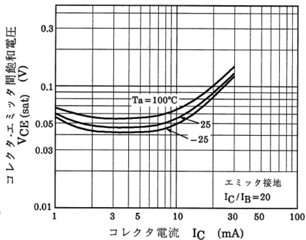
図 13.8 Q2 V_{CE(sat)}-I_C
