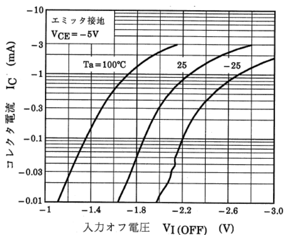
図 13.3 Q1 I_C - V_{I(OFF)}
