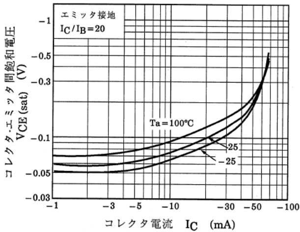
図 13.7 Q1 V_{CE(sat)}-I_C
