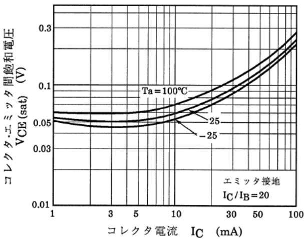
図 13.8 Q2 V_{CE(sat)}-I_C
