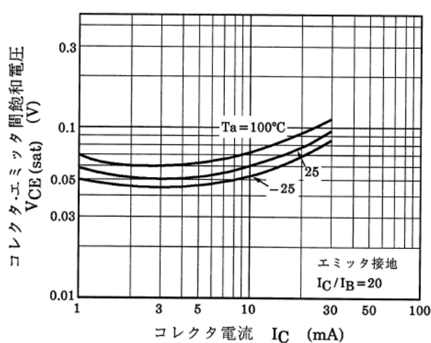
図 13.8 Q2 V_{CE(sat)}-I_C
