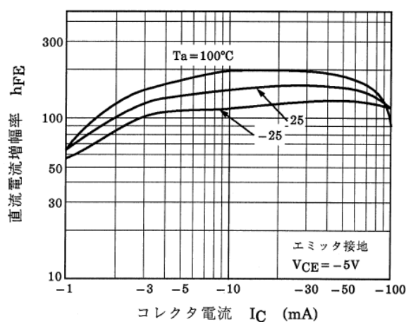
図 13.6 Q2 h_{FE} - I_C
