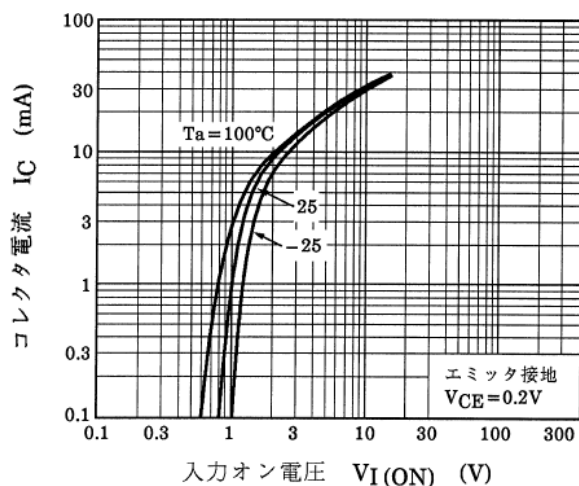
図 13.1 Q1 I_C - V_{I(ON)}
