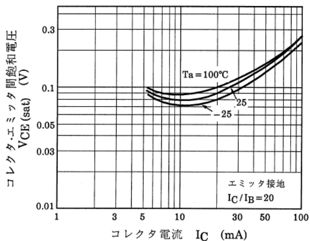
図 13.7 Q1 V_{CE(sat)}-I_C
