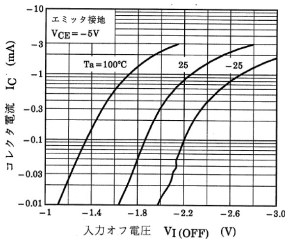
図 13.3 Q1 I_C - V_{I(OFF)}
