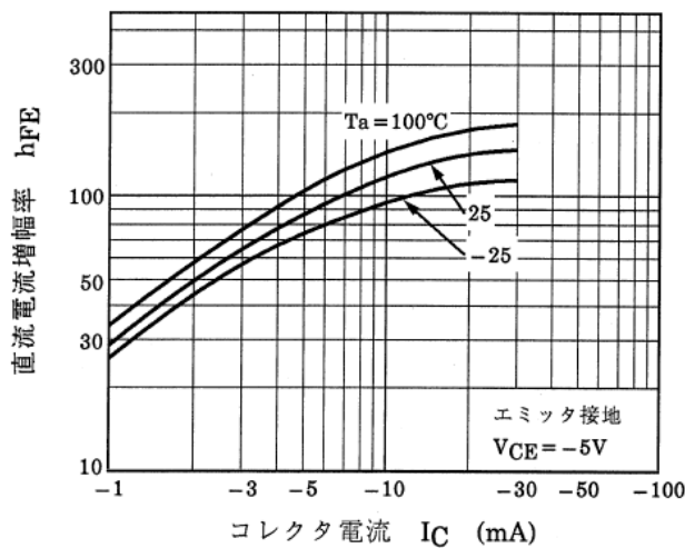
図 10.9 RN2909 h_{FE}-I_C
