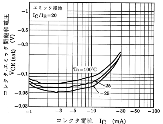
図 10.12 RN2909 V_{CE(sat)}-I_C
