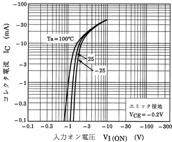
図 10.1 RN2907 I_C - V_{I(ON)}
