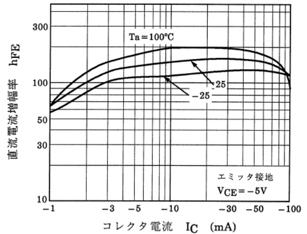
図 10.8 RN2908 h_{FE}-I_C
