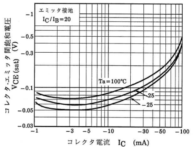
図 10.10 RN2907 V_{CE(sat)}-I_C
