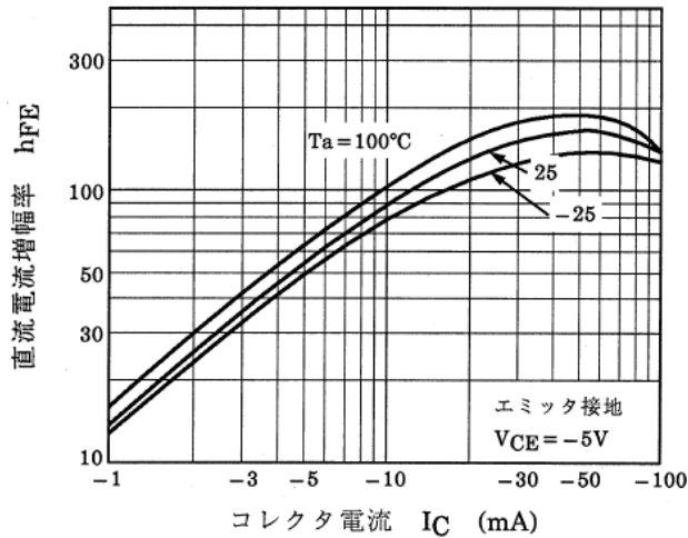
図 10.7 RN2907 h_{FE}-I_C
