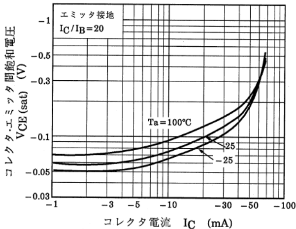
図 10.11 RN2908 V_{CE(sat)}-I_C
