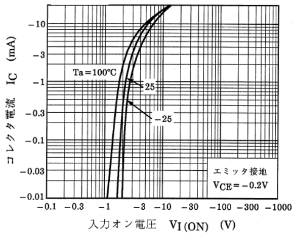
図 10.3 RN2909 I_C - V_{I(ON)}
