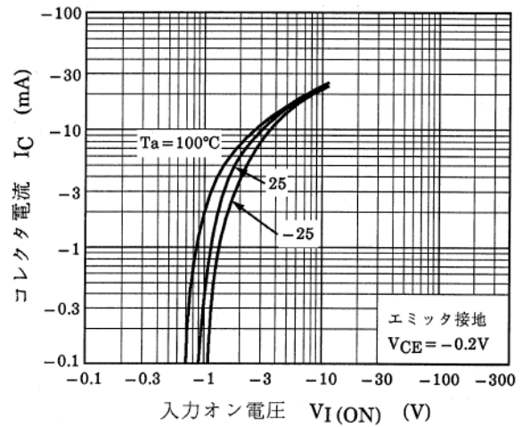
図 10.2 RN2908 I_C - V_{I(ON)}
