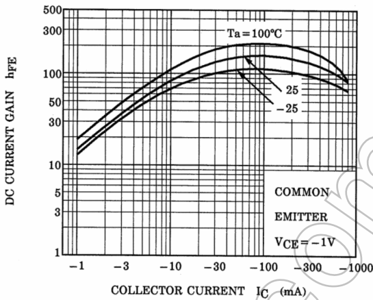
Fig. 9.21 RN2427 h FE -I C
