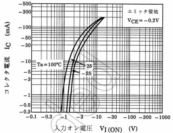
図 9.8 RN2424 I_C - V_{I(ON)}
