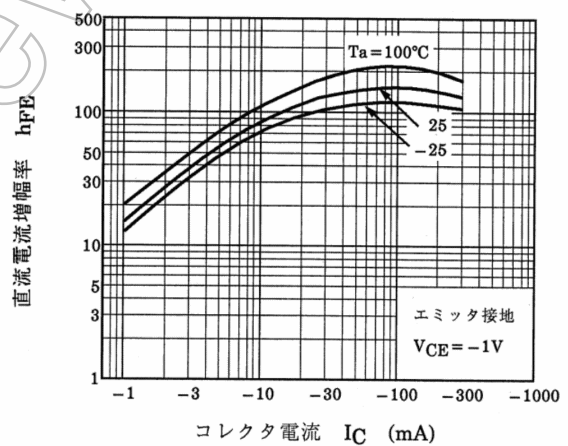
図 9.12 RN2424 h_{FE} - I_C
