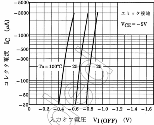
図 9.20 RN2427 I C -V I(OFF)
