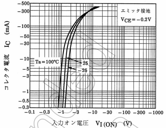
図 9.2 RN2422 I_C - V_{I(ON)}
