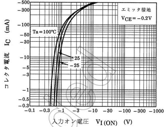
図 9.14 RN2426 I_C-V_{I(ON)}
