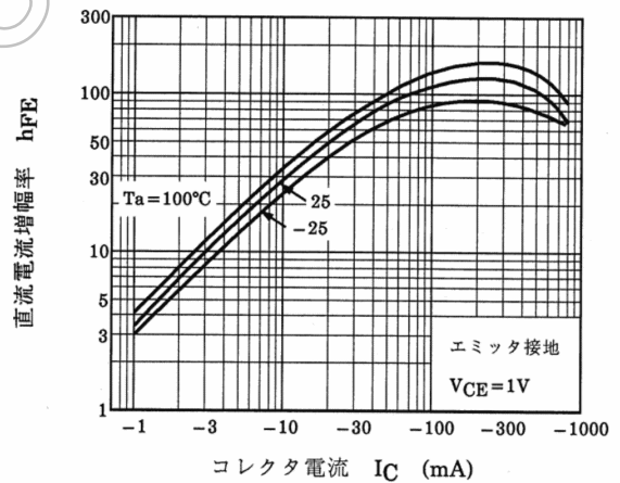
図 9.6 RN2422 h_{FE} - I_C
