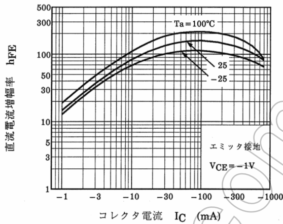
図 9.21 RN2427 hFE-I C
