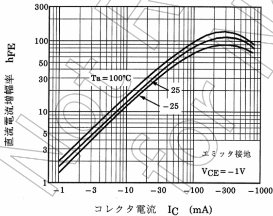
図 9.5 RN2421 h_{FE} - I_C
