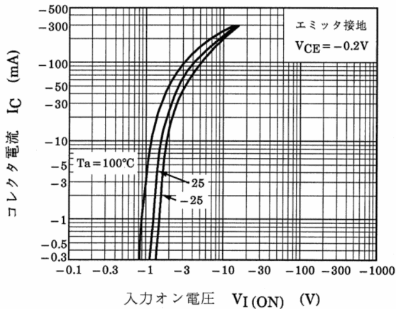
図 9.7 RN2423 I_C - V_{I(ON)}
