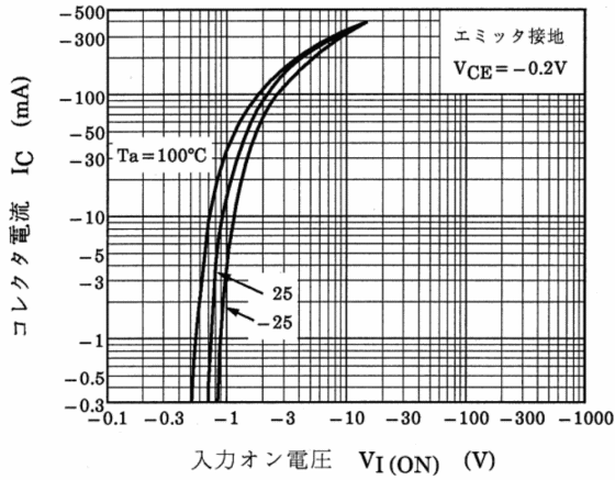
図 9.19 RN2427 I C -V I(ON)
