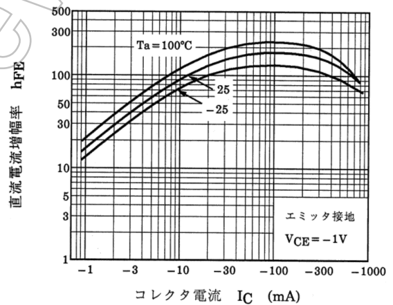
図 9.18 RN2426 h_{FE}-I_C
