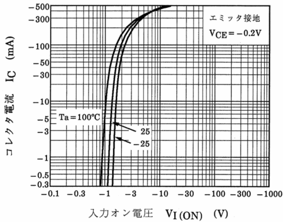
図 9.1 RN2421 I_C - V_{I(ON)}
