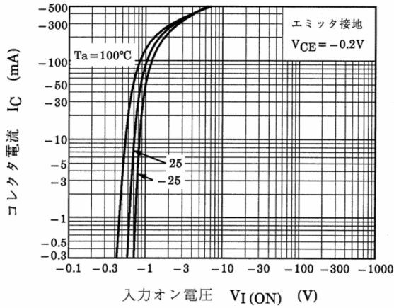
図 9.13 RN2425 I_C-V_{I(ON)}
