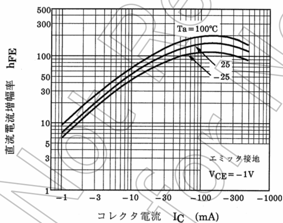
図 9.11 RN2423 h_{FE} - I_C
