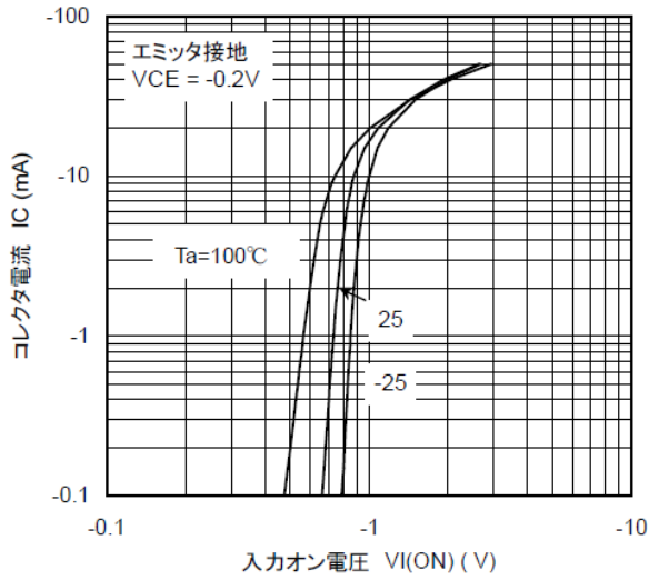
図 10.1 RN2414 IC-VI(ON)
