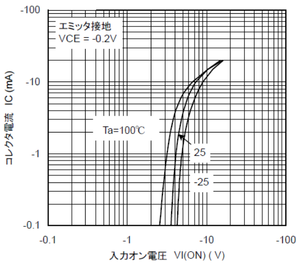
図 10.3 RN2416 IC-VI(ON)
