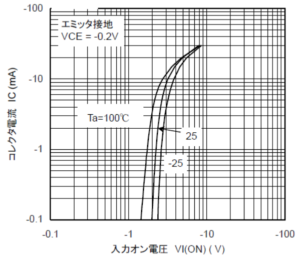
図 10.4 RN2417 IC-VI(ON)
