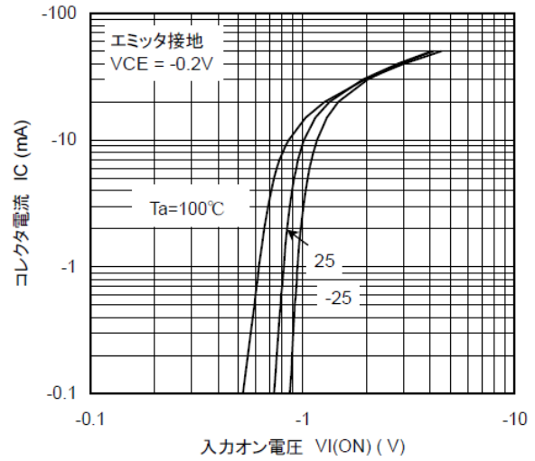
図 10.2 RN2415 IC-VI(ON)
