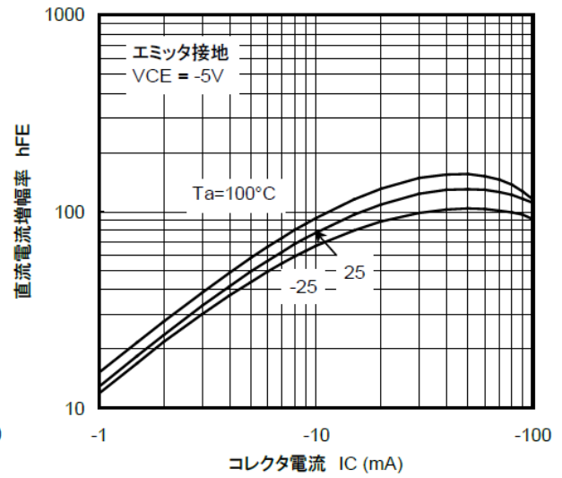
図 10.12 RN2115 h_{FE} - I_C
