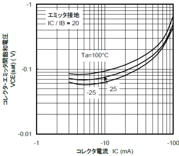
図 10.18 RN2116 V_{CE(sat)}-I_C
