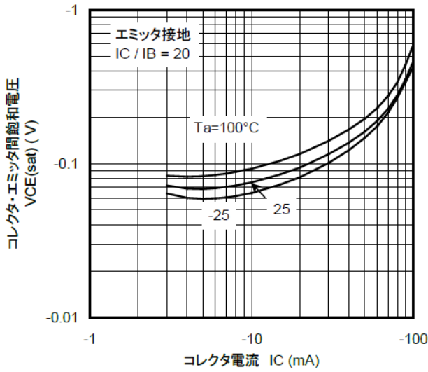
図 10.16 RN2114 V_{CE(sat)}-I_C
