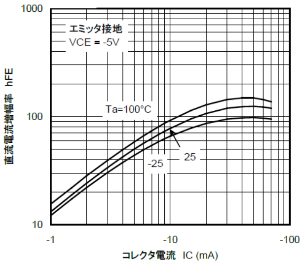
図 10.13 RN2116 h_{FE} - I_C
