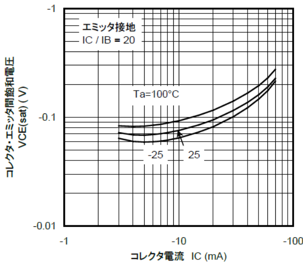
図 10.20 RN2118 V_{CE(sat)}-I_C
