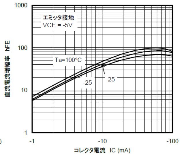
図 10.14 RN2117 h_{FE} - I_C
