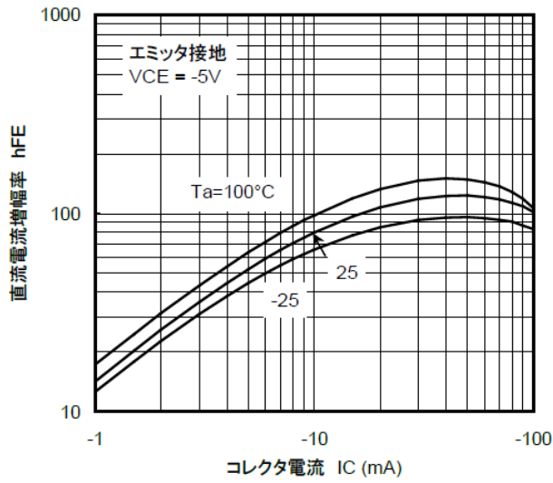
図 10.11 RN2114 h_{FE} - I_C
