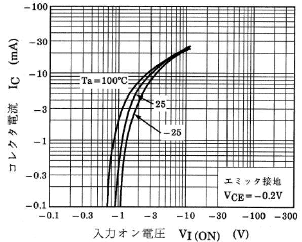
図 10.2 RN2108 I_C - V_{I(ON)}
