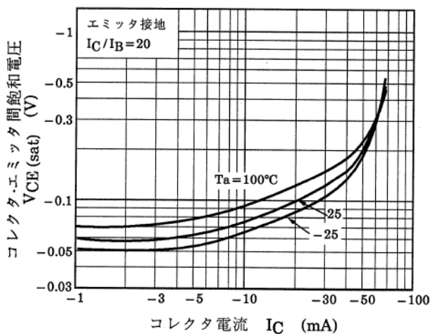
図 10.11 RN2108 V_{CE(sat)}-I_C
