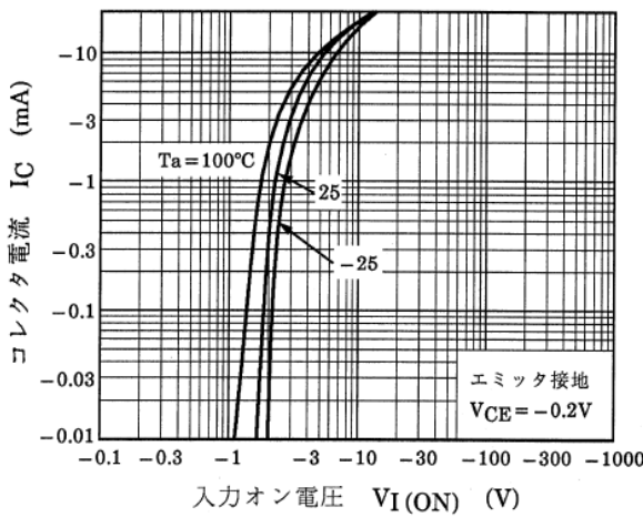
図 10.3 RN2109 I_C - V_{I(ON)}
