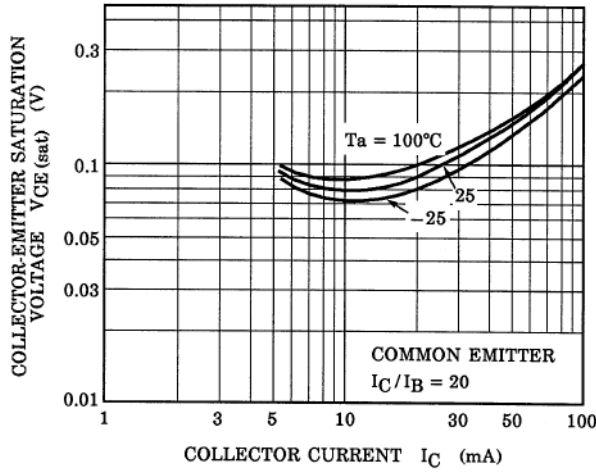
Fig. 10.19 RN1901 V_{CE(sat)}-I_C
