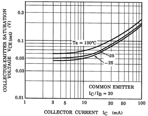
Fig. 10.10 RN1407 V_{CE(sat)}-I_C
