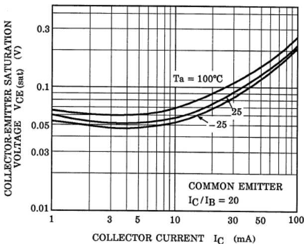
Fig. 10.23 RN1405 V_{CE(sat)} - I_C
