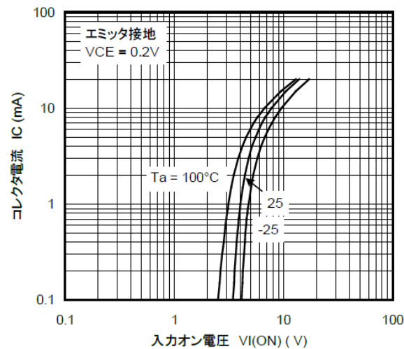
図 10.3 RN1316 I_C - V_{I(ON)}
