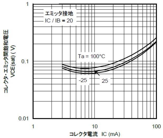
図 10.16 RN1314 V_{CE(sat)} - I_C
