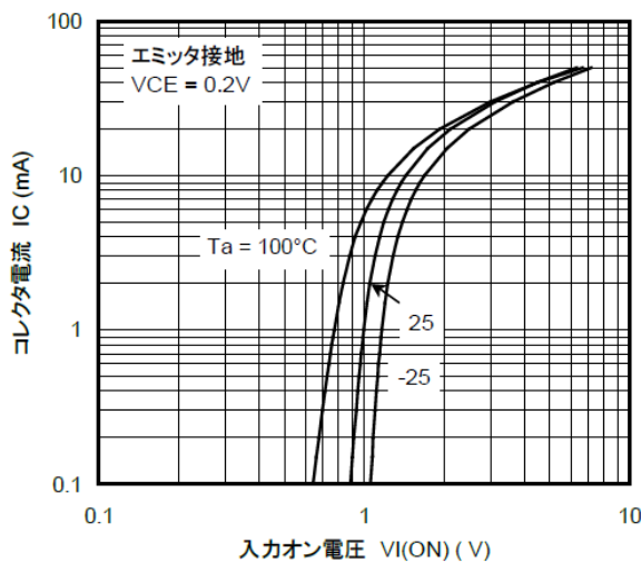
図 10.3 RN1316 I_C - V_{I(ON)}
