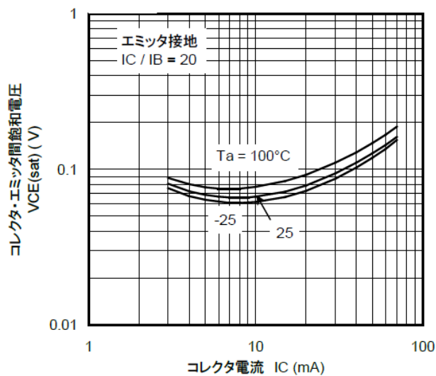
図 10.20 RN1318 V_{CE(sat)} - I_C
