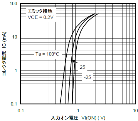
図 10.1 RN1314 I_C - V_{I(ON)}
