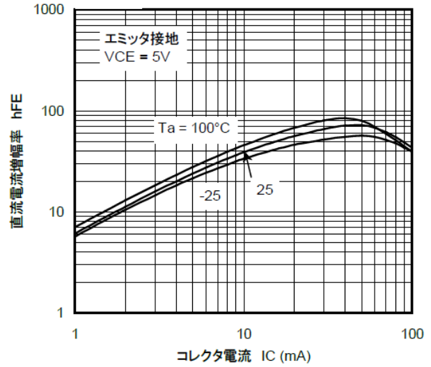
図 10.14 RN1317 h_{FE} - I_C
