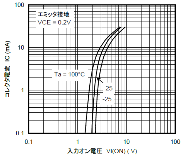
図 10.4 RN1317 I_C - V_{I(ON)}
