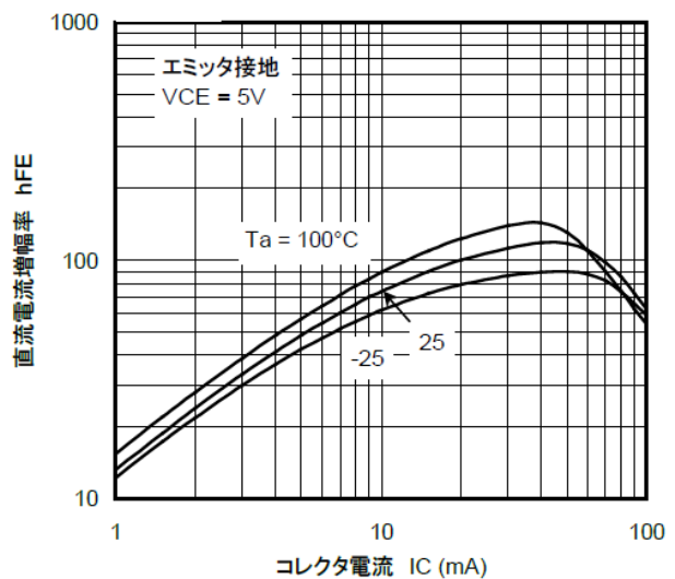
図 10.12 RN1315 h_{FE} - I_C
