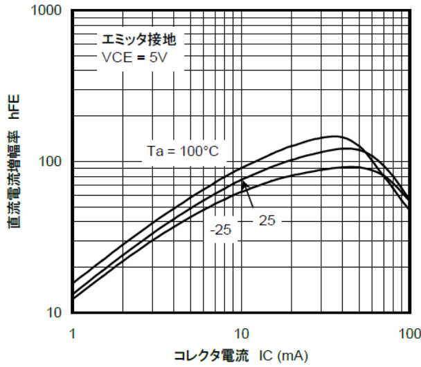
図 10.13 RN1316 h_{FE} - I_C
