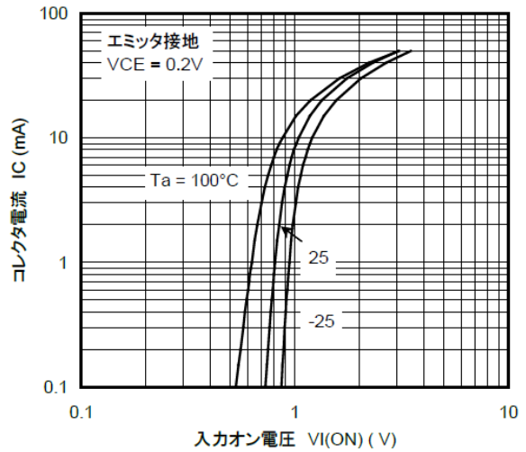
図 10.2 RN1315 I_C - V_{I(ON)}
