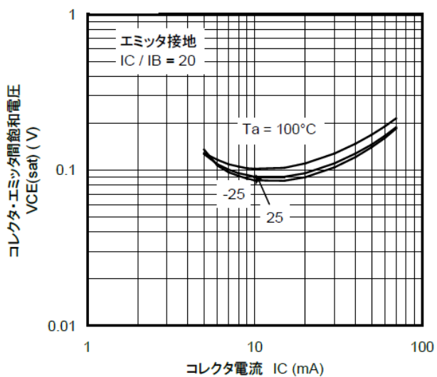
図 10.19 RN1317 V_{CE(sat)} - I_C
