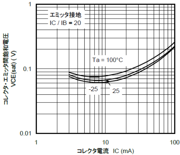
図 10.17 RN1315 V_{CE(sat)} - I_C
