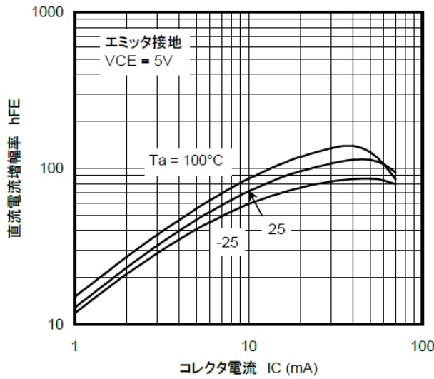
図 10.15 RN1318 h_{FE} - I_C
