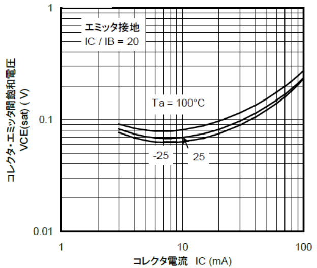
図 10.18 RN1316 V_{CE(sat)} - I_C
