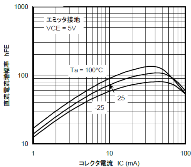
図 10.11 RN1314 h_{FE} - I_C
