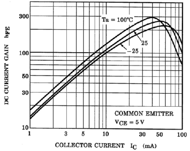
Fig. 10.14 RN1302 h_{FE}-I_C
