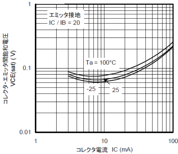
図 10.16 RN1114 V_{CE(sat)} - I_C
