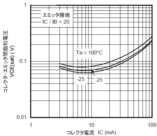
図 10.18 RN1116 V_{CE(sat)} - I_C
