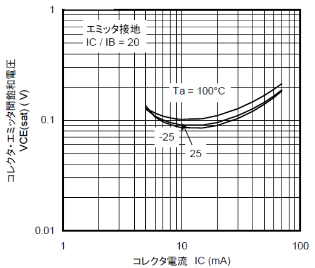
図 10.19 RN1117 V_{CE(sat)} - I_C
