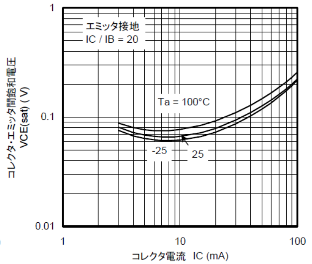
図 10.17 RN1115 V_{CE(sat)} - I_C
