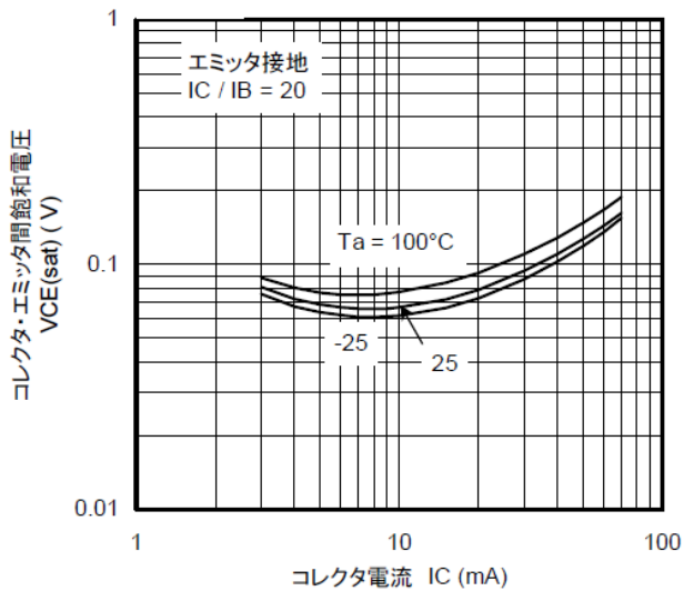
図 10.20 RN1118 V_{CE(sat)} - I_C
