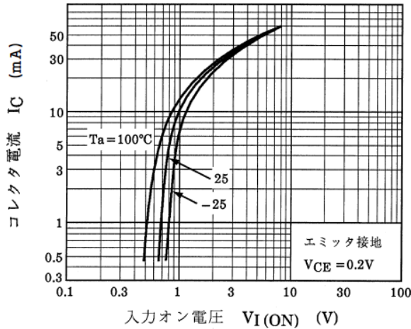
図 9.1 RN1110 I_C - V_{I(ON)}
