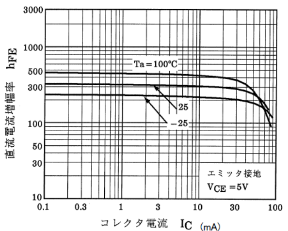
図 9.6 RN1111 h_{FE} - I_C
