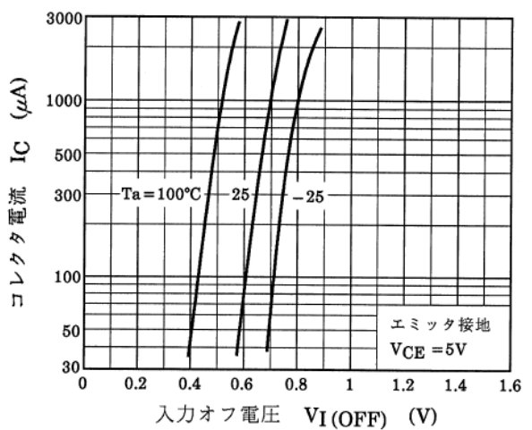
図 9.4 RN1111 I_C - V_{I(OFF)}
