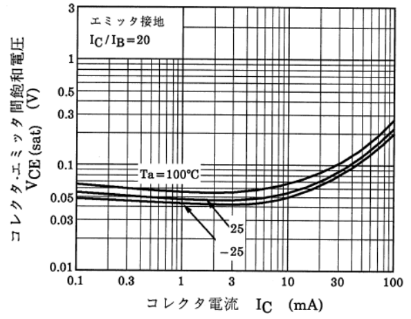
図 9.8 RN1111 V_{CE(sat)}-I_C
