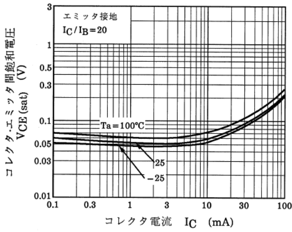
図 9.7 RN1110 V_{CE(sat)}-I_C
