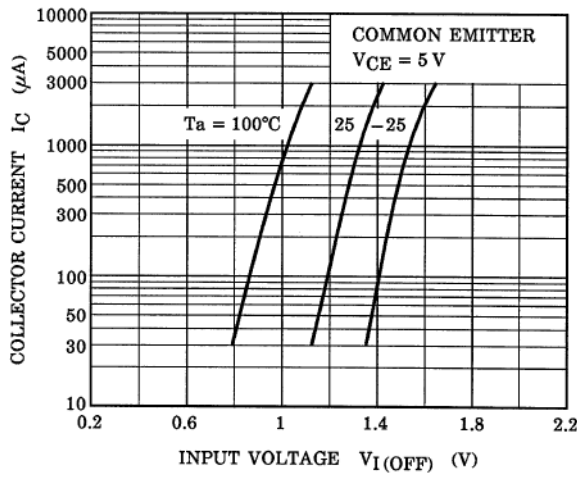
Fig. 10.7 RN1101 I C -V I(OFF)
