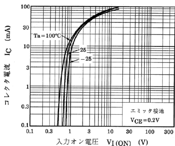
図 10.5 RN1105 I_C - V_{I(ON)}
