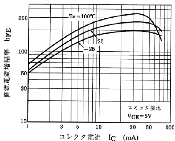
図 10.16 RN1104 h_{FE} - I_C
