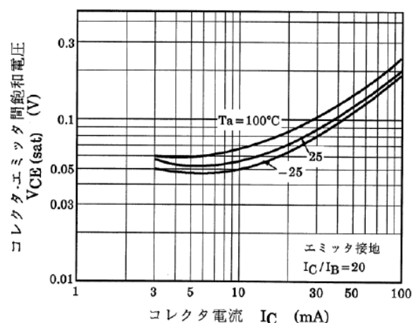
図 10.20 RN1102 V_{CE(sat)}-I_C
