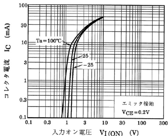
図 10.2 RN1102 I_C - V_{I(ON)}
