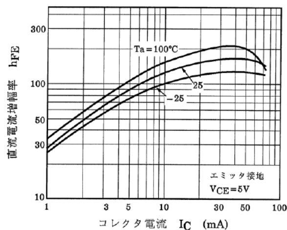
図 10.15 RN1103 h_{FE} - I_C
