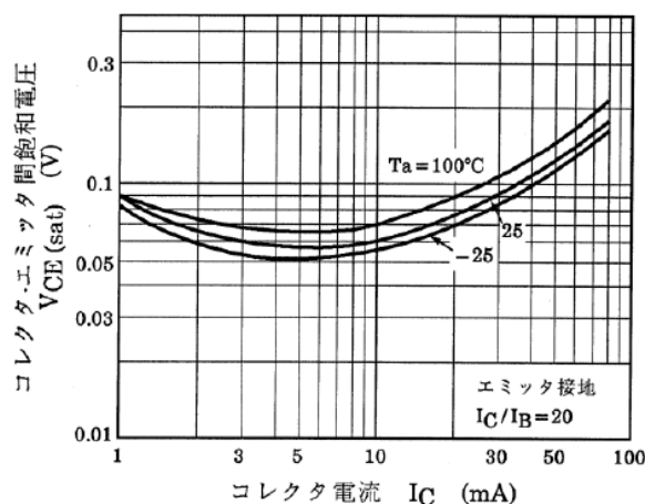
図 10.21 RN1103 V_{CE(sat)}-I_C
