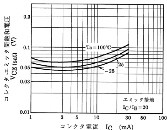
図 10.22 RN1104 V_{CE(sat)}-I_C
