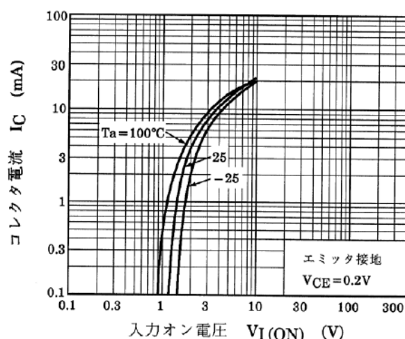
図 10.4 RN1104 I_C - V_{I(ON)}
