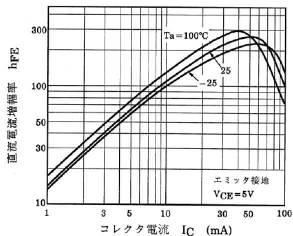
図 10.14 RN1102 h_{FE} - I_C
