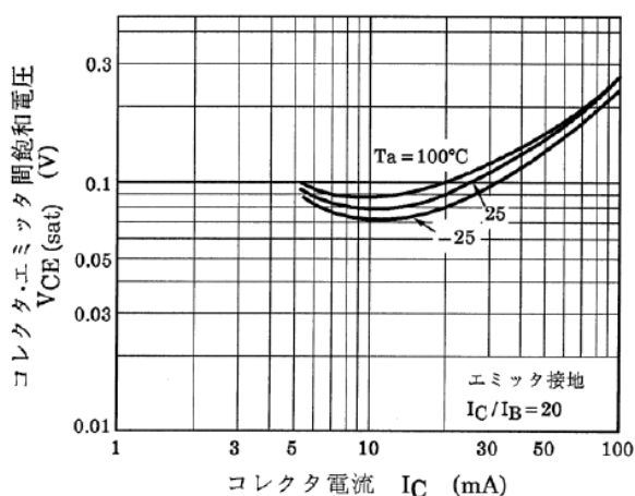
図 10.19 RN1101 V_{CE(sat)}-I_C
