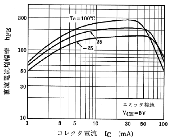
図 10.18 RN1106 h_{FE} - I_C
