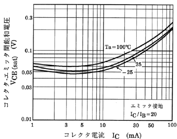
図 10.23 RN1105 V_{CE(sat)}-I_C
