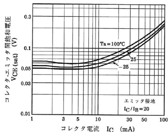
図 10.24 RN1106 V_{CE(sat)}-I_C
